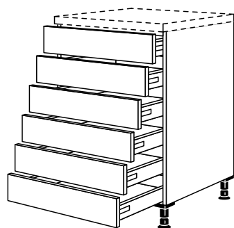
U6S*-M MAXI base unit
